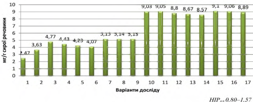
Рис. 1. Вміст леггемоглобіну в бульбочках сої у фазу цвітіння за дії різних норм гербіциду Фабіан, регулятора росту рослин Регоплант і мікробіологічного препарату Ризобофіт (середнє за роки досліджень)
